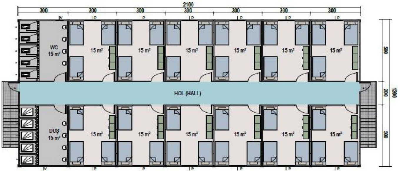
Üst Kat Planı - First Floor (252m 2 )
